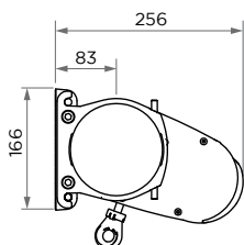
Ambre et Ambre Lux - Pose FACE avec Treuil
