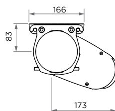
Ambre et Ambre Lux - Pose PLAFOND sans équerre
