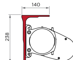
Ambre et Ambre Lux - Pose PLAFOND avec équerre
