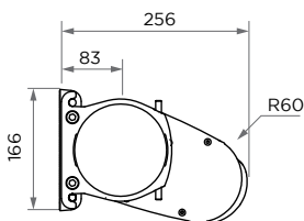
Ambre et Ambre Lux - Pose FACE
