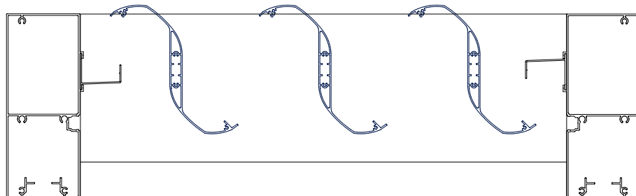
ÉVACUATION DE L'EAU DE PLUIE La position permettra l'évacuation de l'eau de pluie vers les gouttières.
